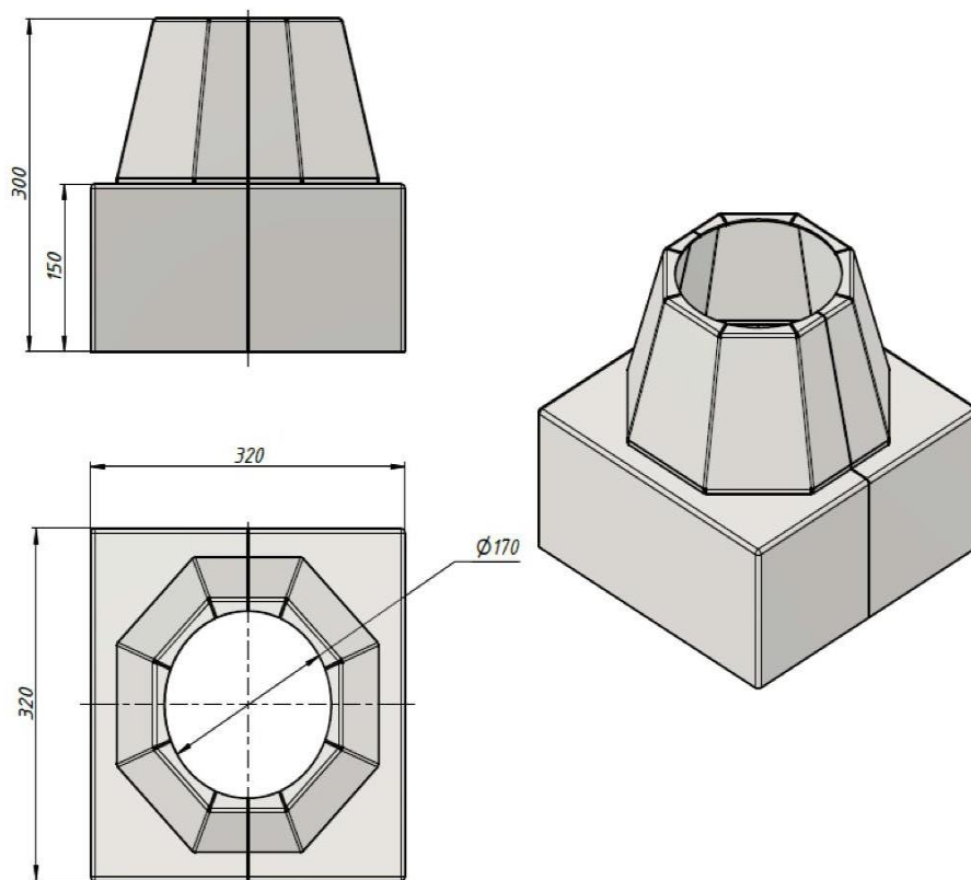
Мал.1 Габаритні і приєднувальні розміри
