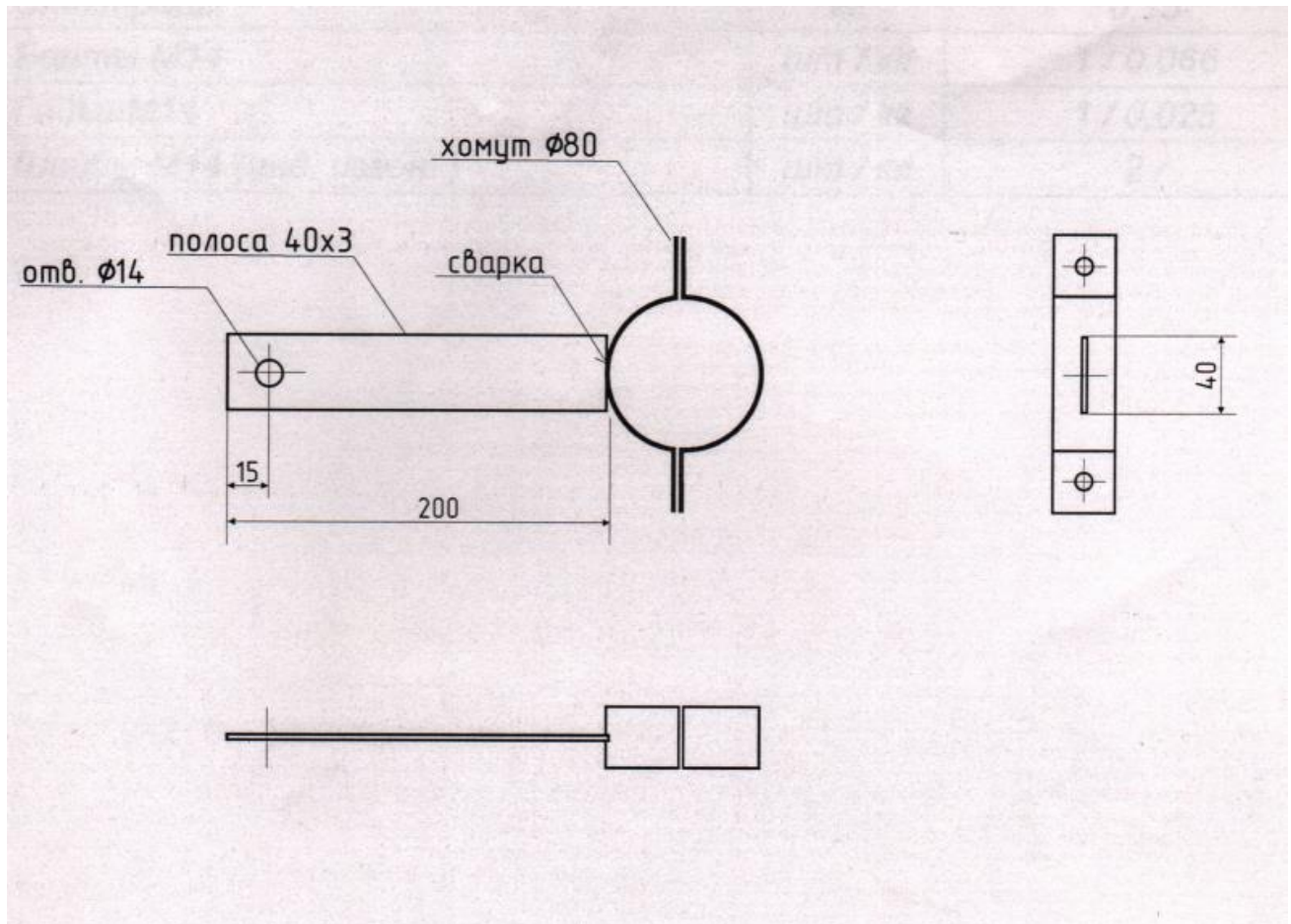
Мал.1 Габаритні і приєднувальні розміри
