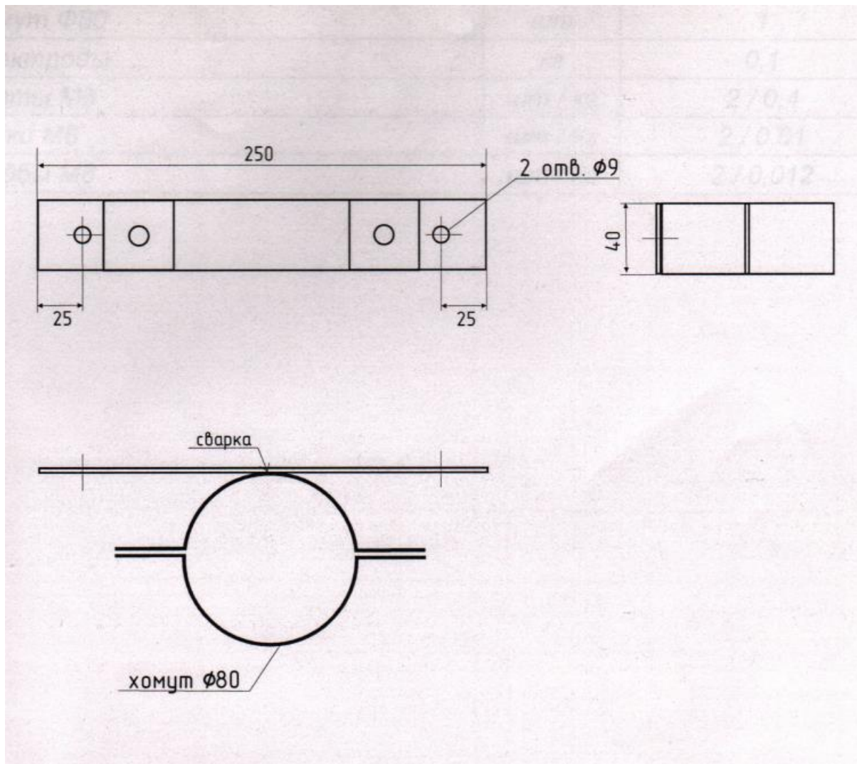
Мал.1 Габаритні і приєднувальні розміри
