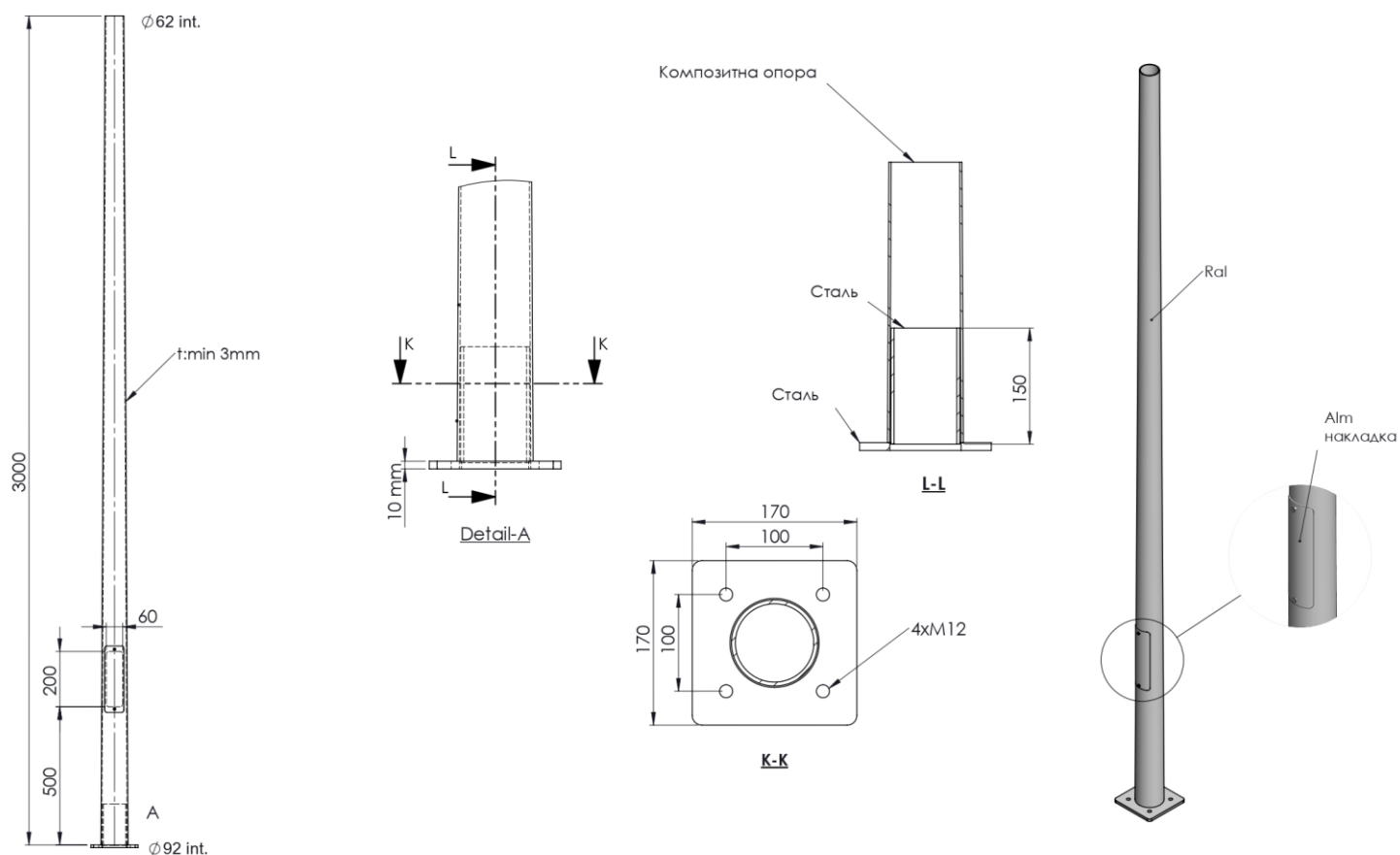
Мал.1 Габаритні і приєднувальні розміри
