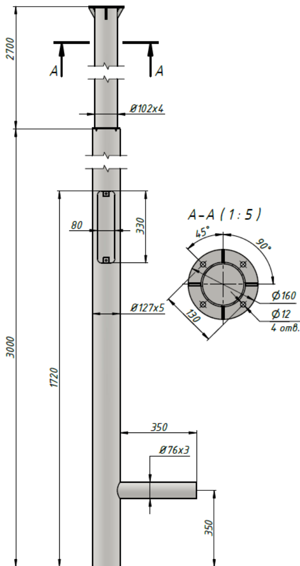
Мал.1 Габаритні і приєднувальні розміри
