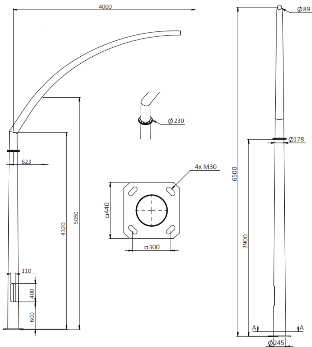
Мал.1 Габаритні і приєднувальні розміри
