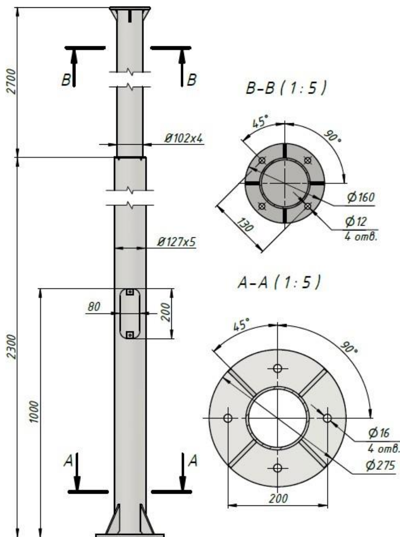
Мал.1 Габаритні і приєднувальні розміри
