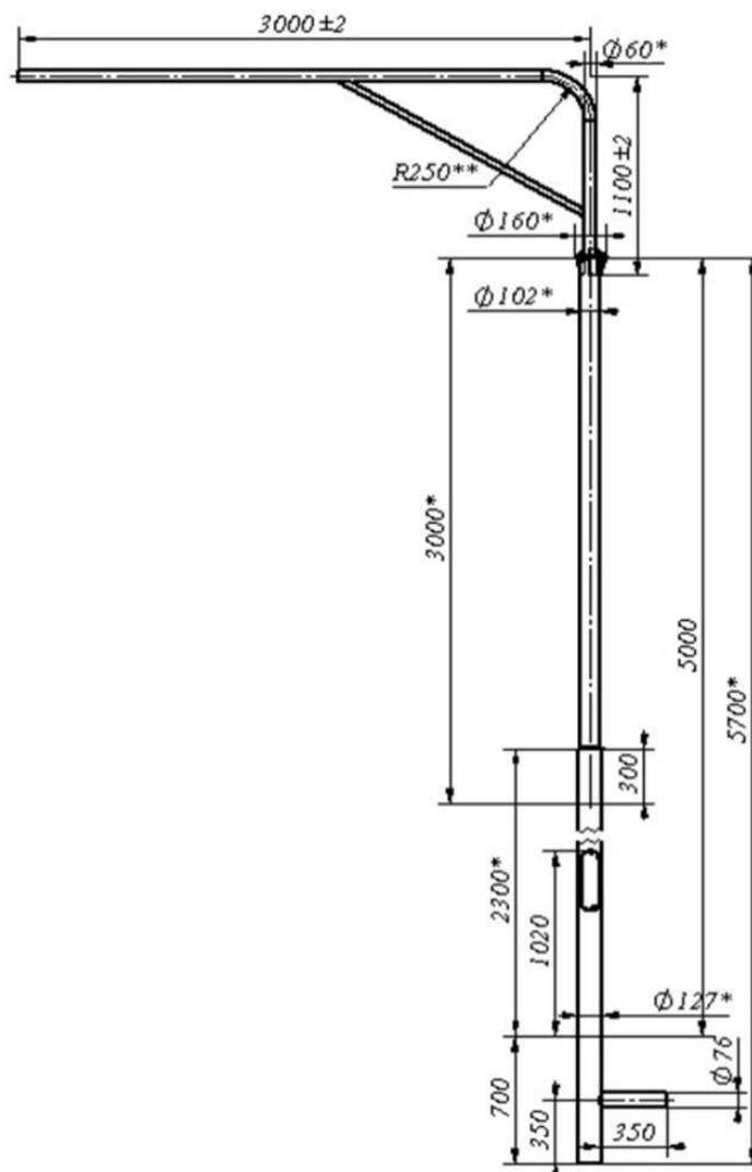
Мал.1 Габаритні і приєднувальні розміри
