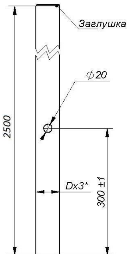
Мал.1 Габаритні і приєднувальні розміри
