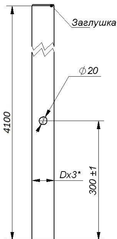
Мал.1 Габаритні і приєднувальні розміри
