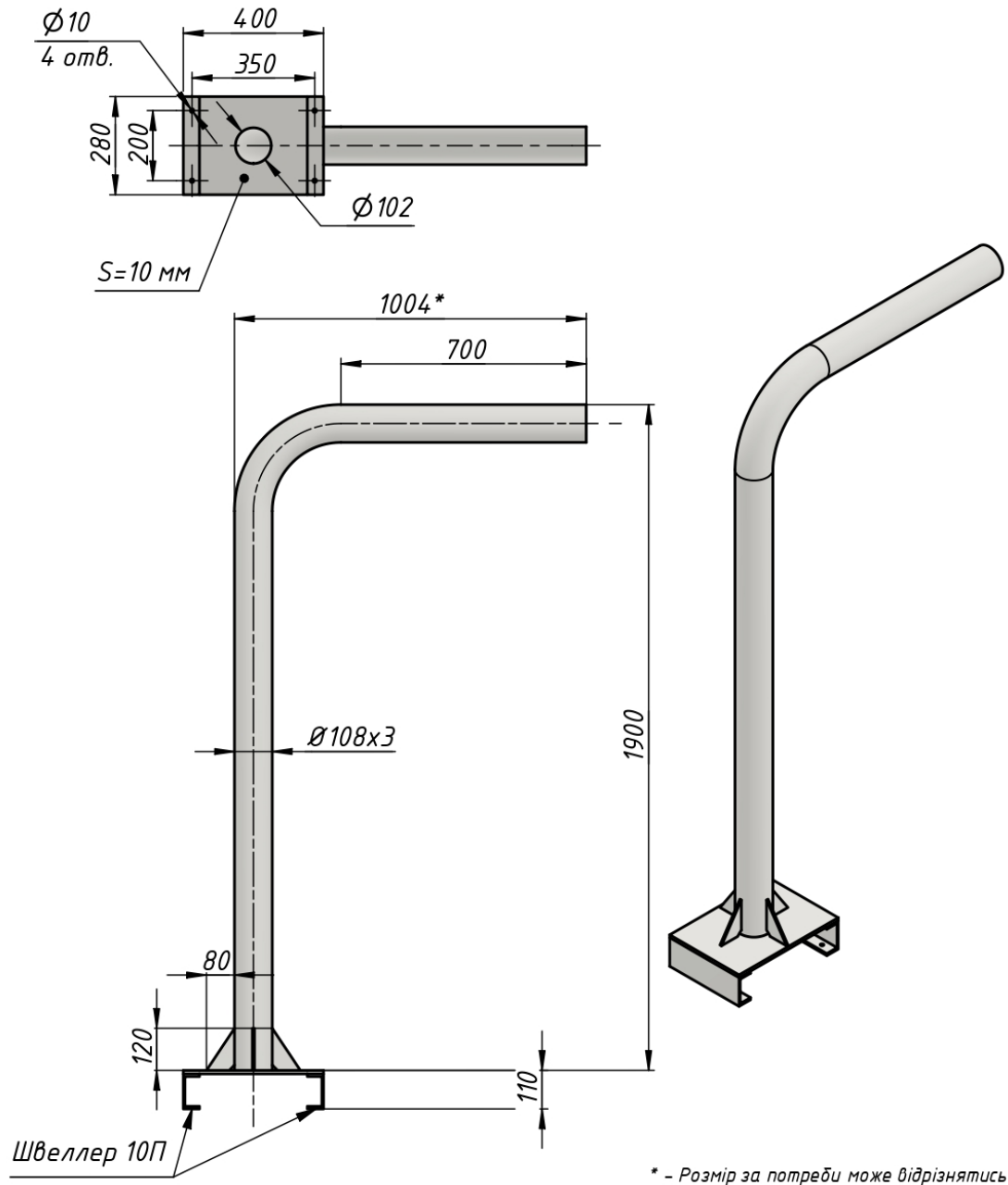
Мал.1 Габаритні і приєднувальні розмір
