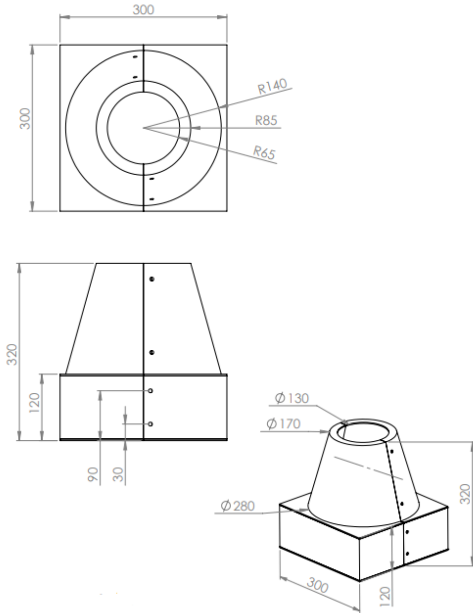
Мал.1 Габаритні і приєднувальні розміри
