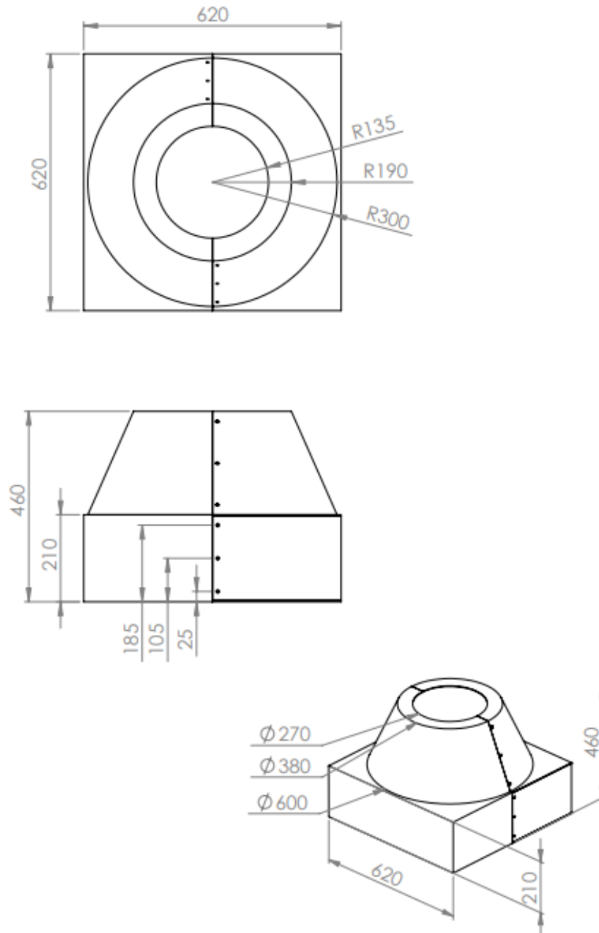
Мал.1 Габаритні і приєднувальні розміри
